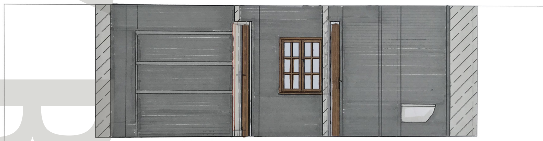
B-B'
